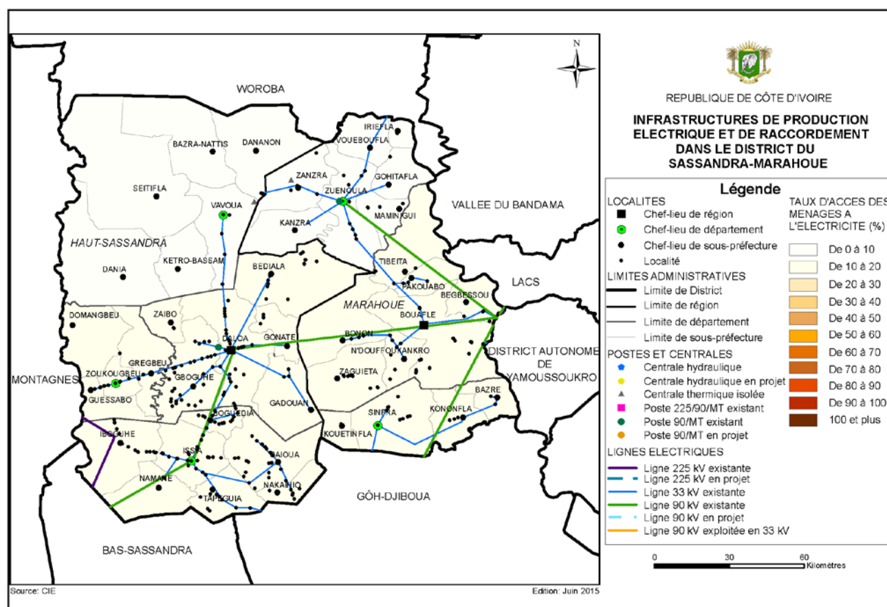
Carte 54 : Infrastructures de production électrique et de raccordement
