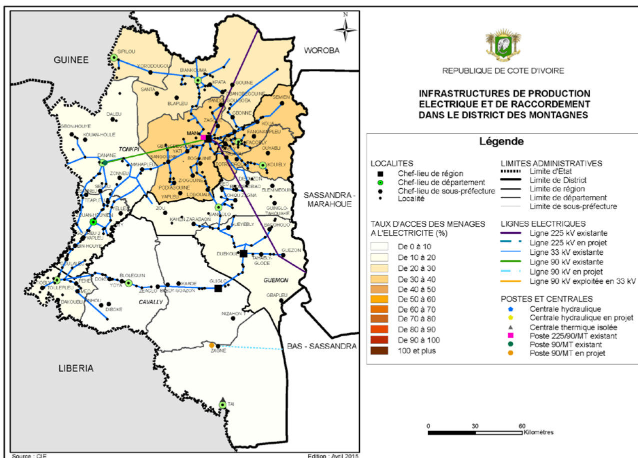
Carte 52 : Infrastructures de production électrique et raccordements
